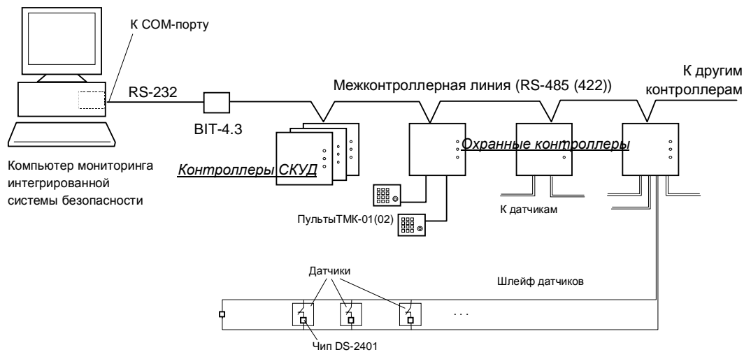
Рис.1. Схема организации системы сигнализации на базе контроллеров серий TSS-201 и TSS-203
