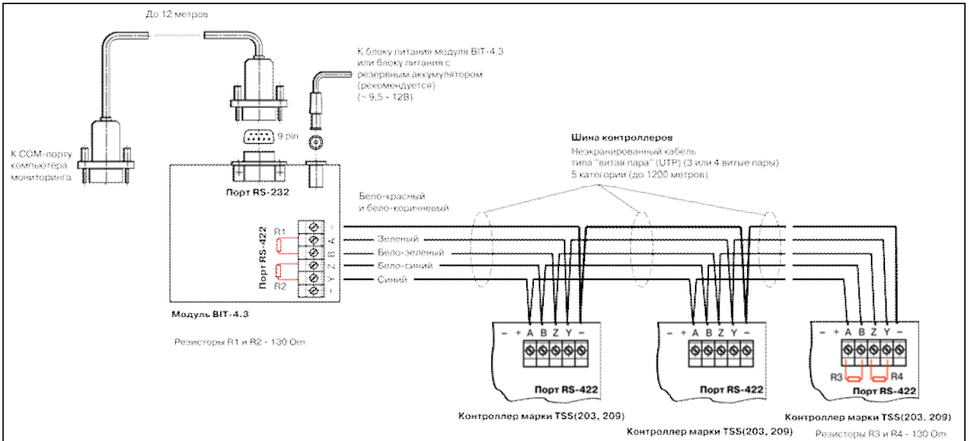
Рис. 5(а). Подключение межконтроллерной линии контроллеров TSS к серверу СКУД
